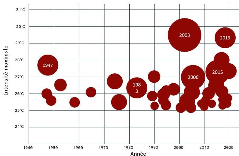
Vagues de chaleurs observées en France de 1947 à 2022 (Météo France)
